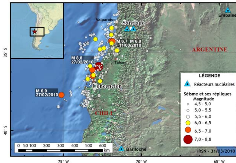
Figure 1 : Localisation du séisme chilien du 27 février 2010 et de ses répliques au 29 mars 2010.
