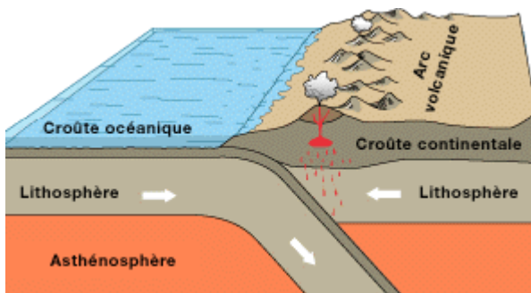
Figure 2 : Subduction d'une plaque océanique sous une plaque continentale
