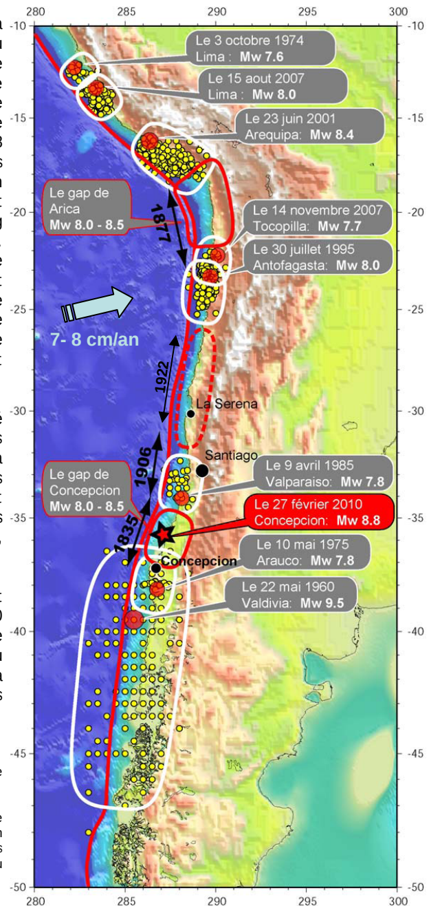
Figure 3 : Zones de rupture des principaux séismes de la subduction chilienne (d'après Ch. Vigny, ENS).
