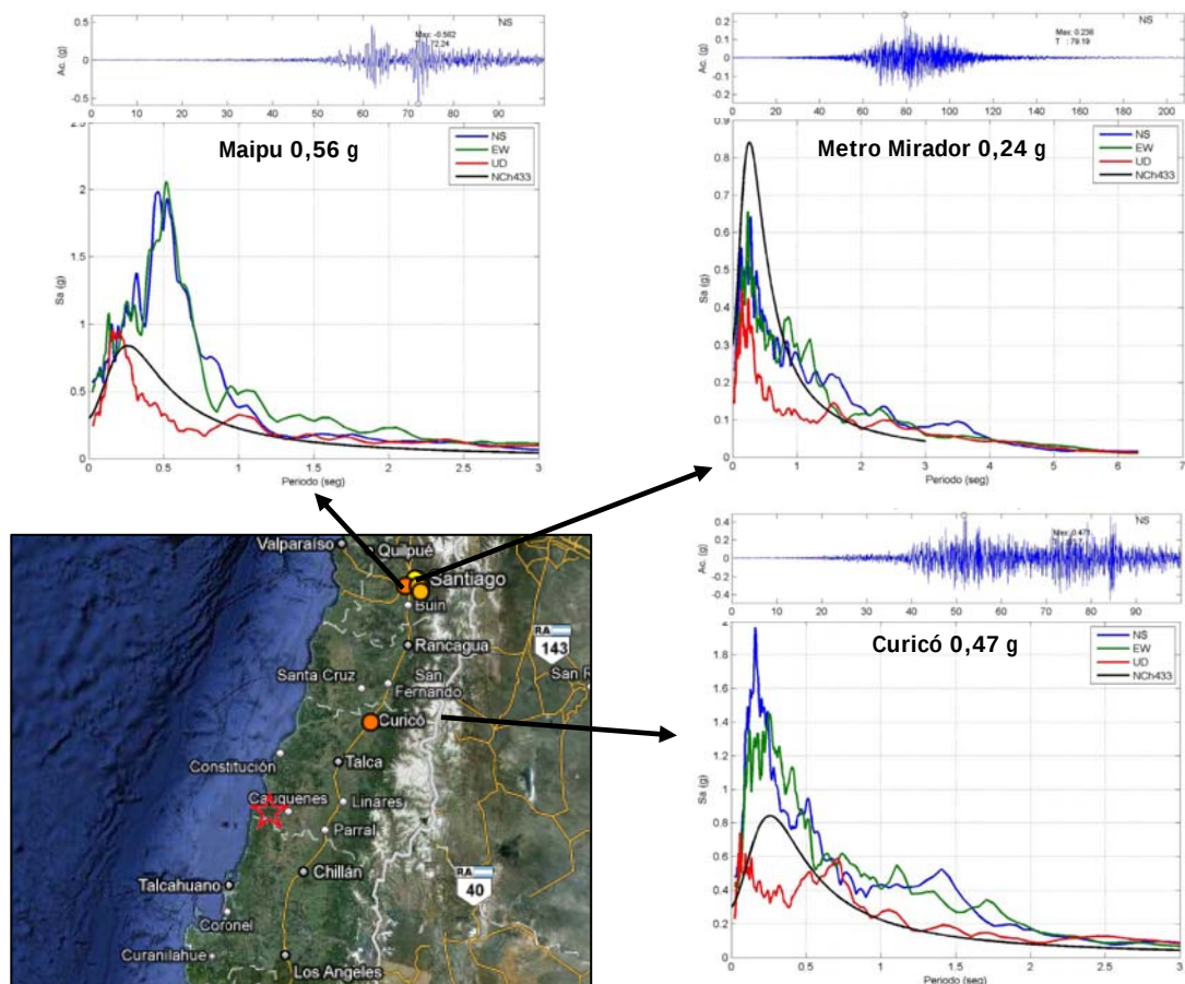
Figure 4 : Accélérations du sol mesurées par différentes stations sismologiques du réseau chilien. Le signal sismique enregistré est représenté en bleu. Les spectres de réponse élastique correspondants (accélérations maximales d'un oscillateur en fonction de sa période propre de vibration) sont comparés à ceux préconisés par la norme parasismique NCh433 en vigueur (courbes noires). Sources : département d'ingénierie civile de l'Université du Chili et www.strongmotioncenter.org .
