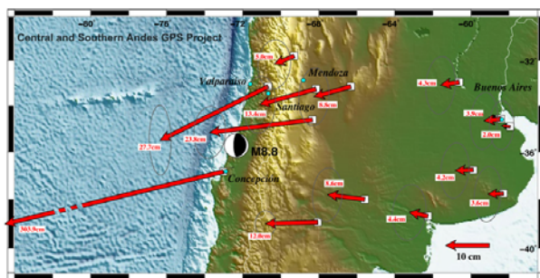
Figure 6 : Déplacement en surface de sites de référence positionnés par GPS, dû au séisme du 27 février 2010. Les flèches rouges indiquent que l'ensemble de cette région d'Amérique du Sud a subi une déformation vers l'Ouest avec un déplacement maximum de 3 mètres mesuré à Concepción (James Foster et Ben Brooks - University Hawaii).
